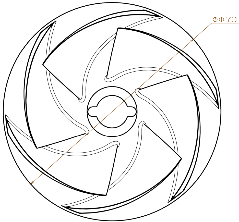
正面图 (1:1)
