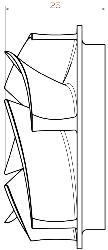
右侧面图 (1:1)
